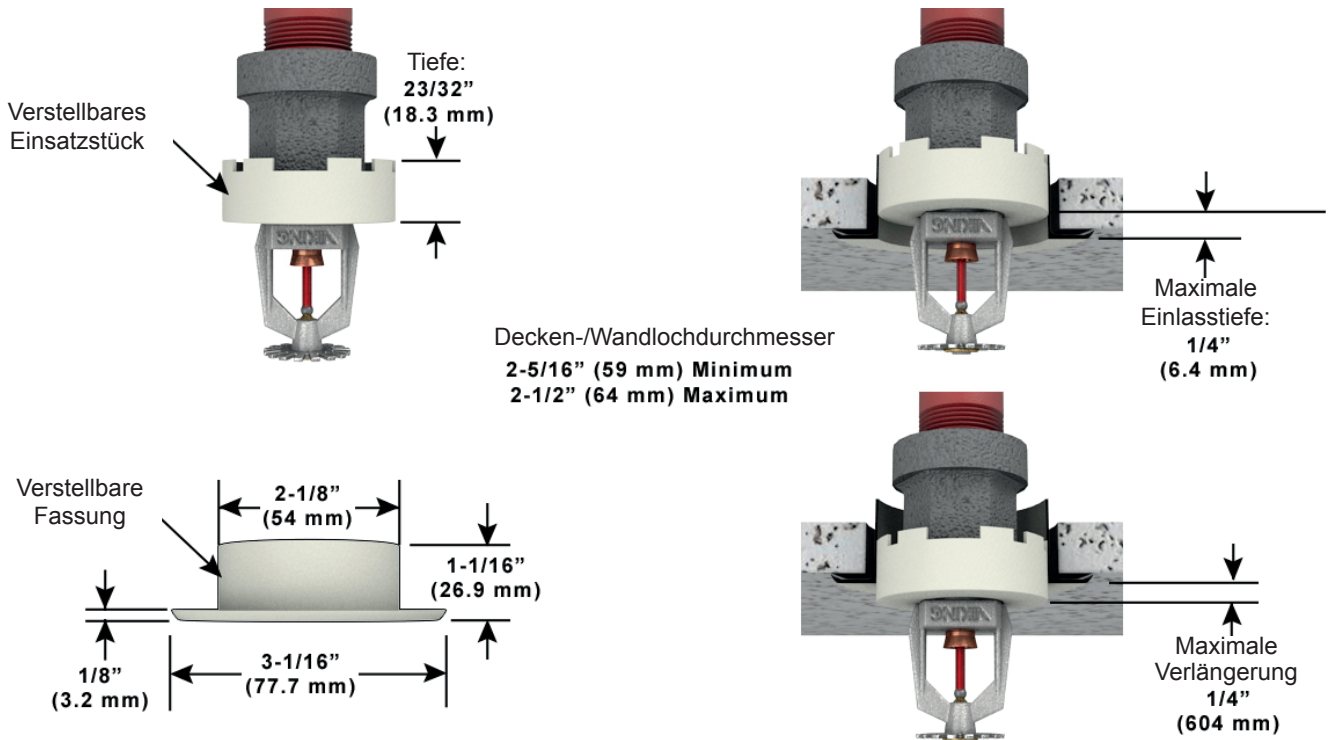
Abbildung 5 : Einbau einer verstellbaren Rosette Micromatic Modell F-1 mit 21 mm Gesamtverstellbereich
