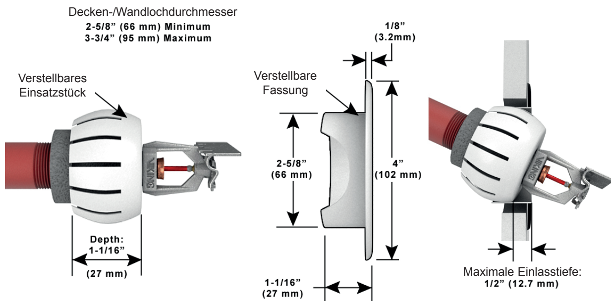
Abbildung 6 : Einbau einer zurückgesetzten Rosette Modell G-1 mit bis zu 12,7 mm Verstellbereich
