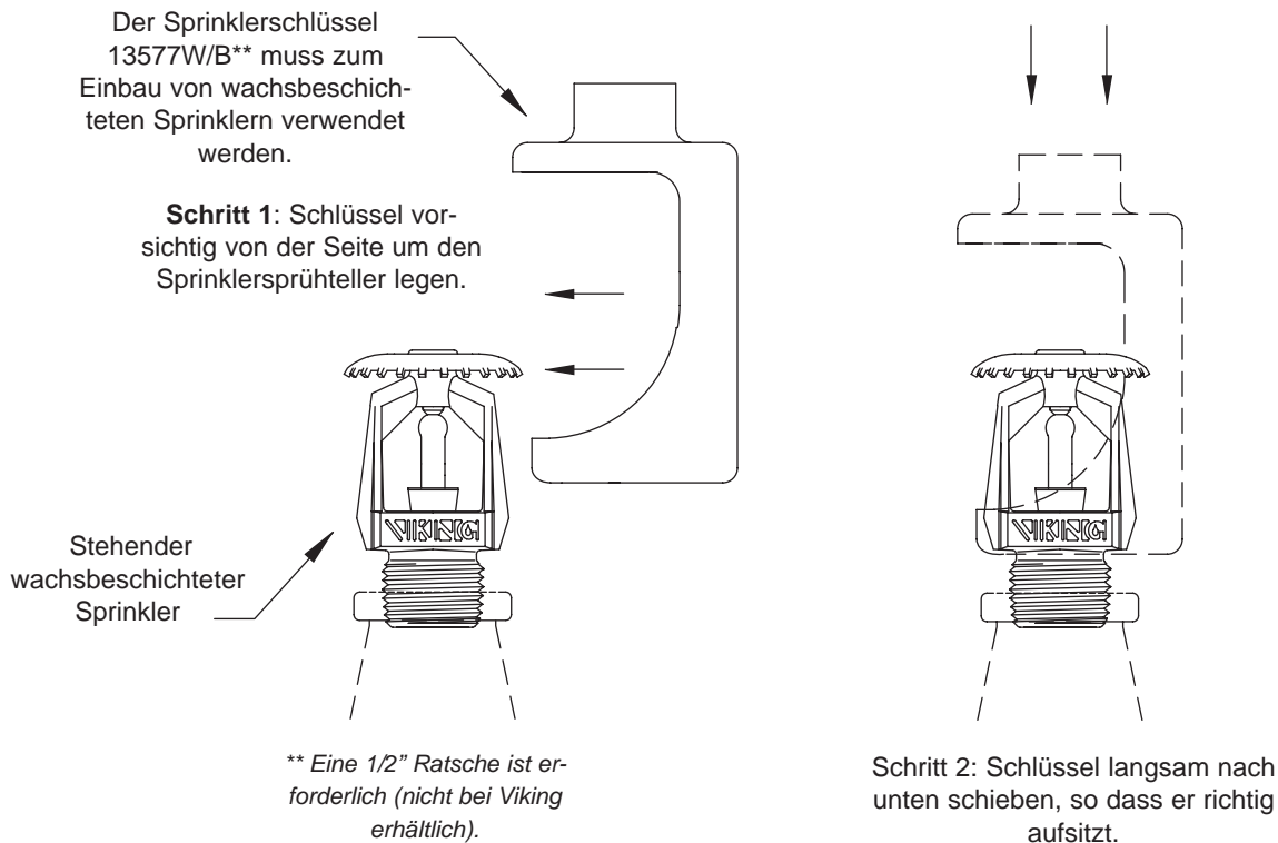
Abbildung 2: Schlüssel 13577W/B für wachsbeschichtete Sprinkler
