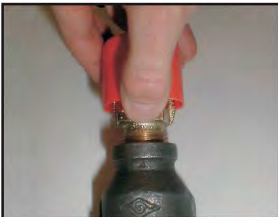
Figure 3 : Enlèvement du capuchon d'un sprinkleur debout.
