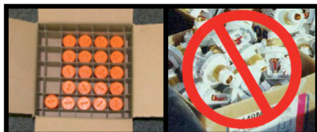
CORRECT (Sprinkleurs protégés par capuchon) INCORRECT (Les capuchons manquent)
