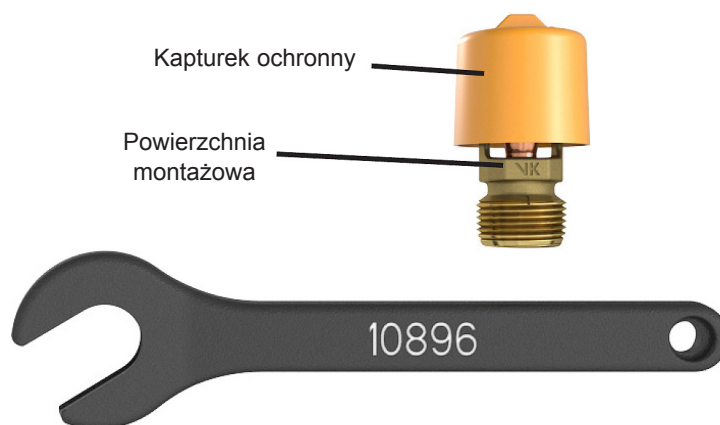
Rysunek nr 1: Klucz standardowy numer 10896W/B
