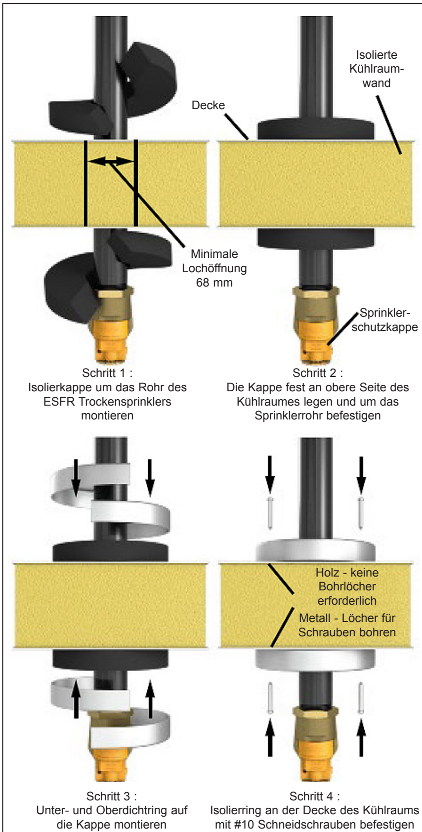
Abbildung 1 : Einbau von Isolierkappen mit gerieftem ESFR Sprinkler
