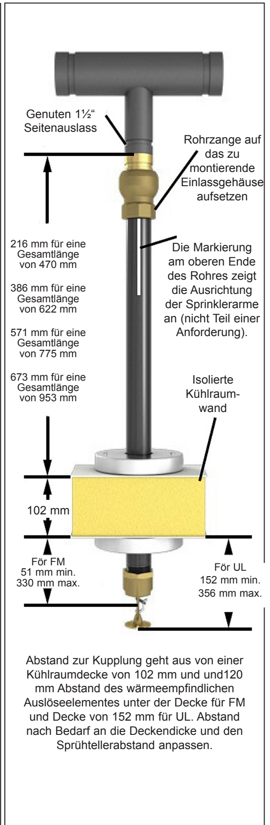
Abbildung 2: Montierter genuten hängender ESFR Trockensprinkler VK504
