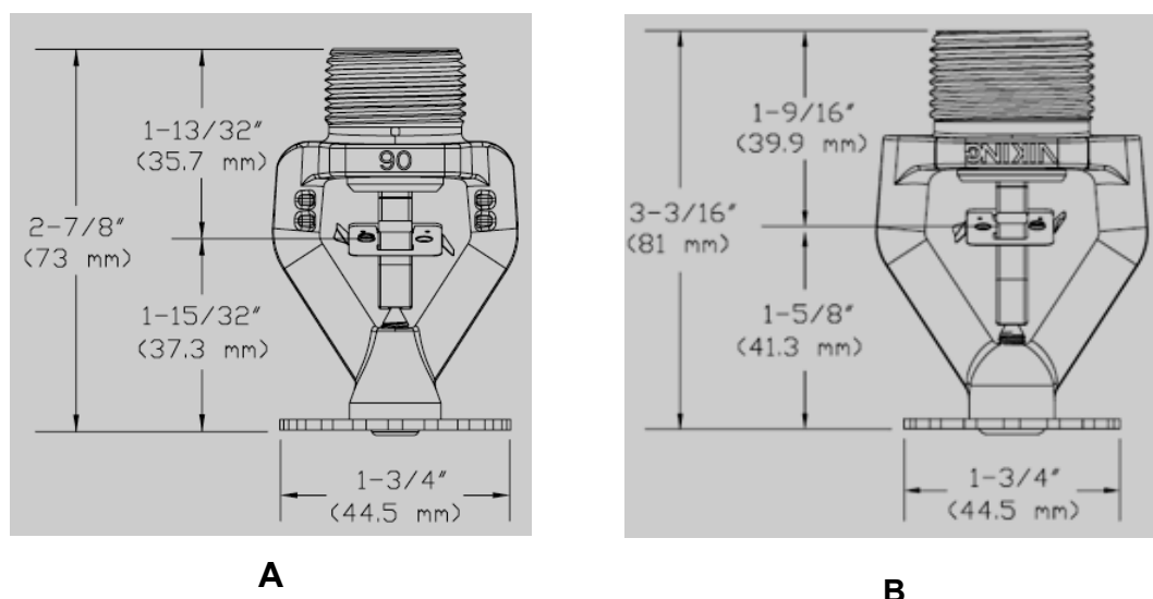
Rys. 3 Wymiary tryśkacza typu VK503 (rys. A) i typu VK506 (rys. B)
